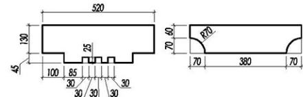
Е - Е
