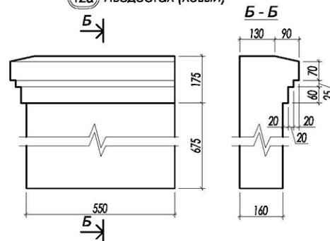
Вид - I
