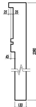
Ж - Ж
