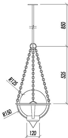
Фонарь подвесной
