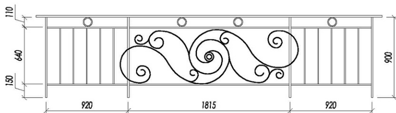
Ограждение террасы
