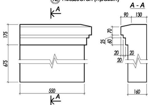
12 Пьедестал (правый)
